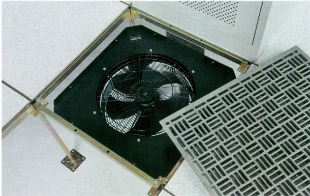
Fan Unit
